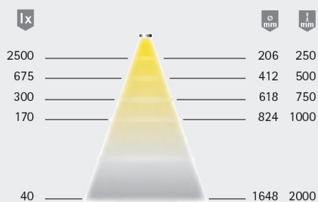
Diagrama de distribución luminosa / 45°
